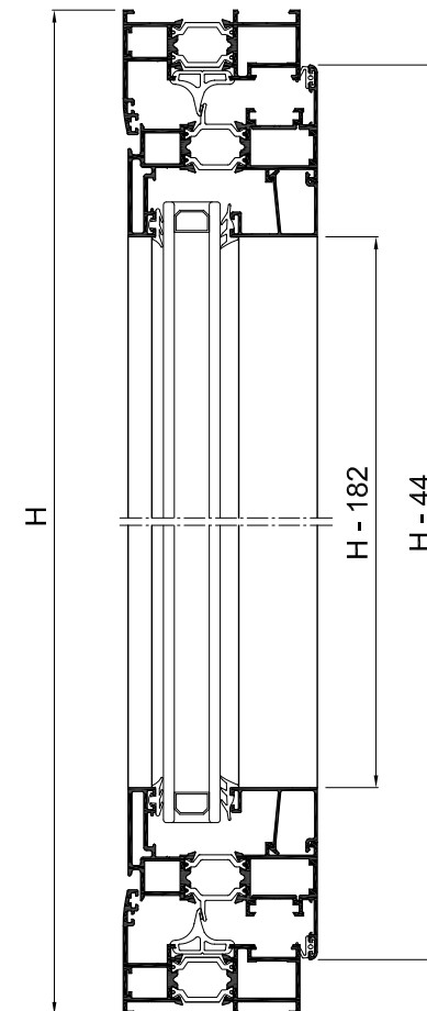
Sección B-B'
