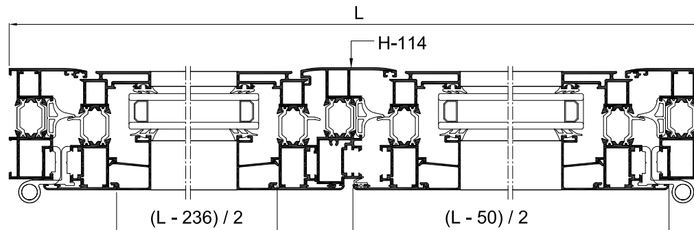
Sección A-A'
